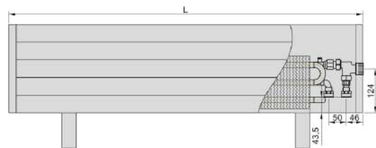
APATINIS PAJUNGIMAS
