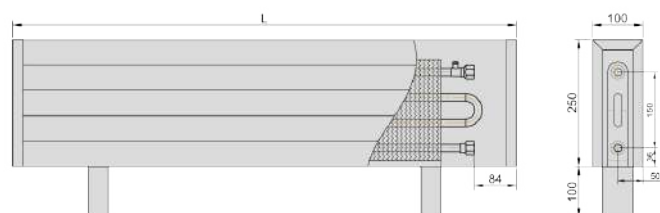
ŠONINIS PAJUNGIMAS
