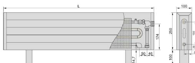
APATINIS PAJUNGIMAS
