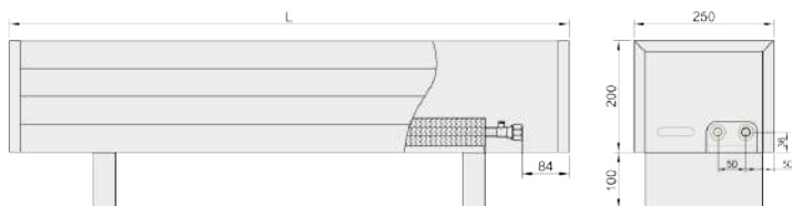
ŠONINIS PAJUNGIMAS
