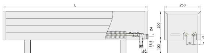
APATINIS PAJUNGIMAS
